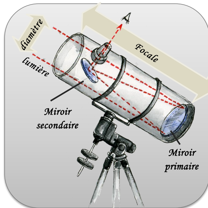
Dans un télescope de type Newton
