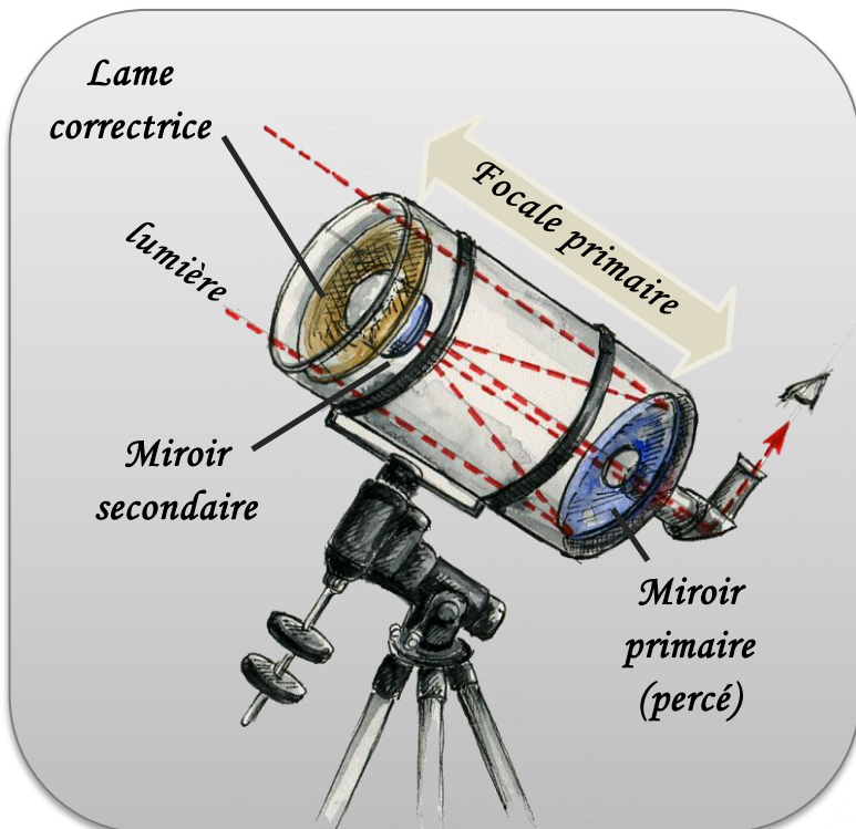
Dans un télescope de type Schmidt-Cassegrain
